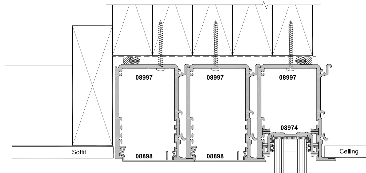
SECTION A-A
