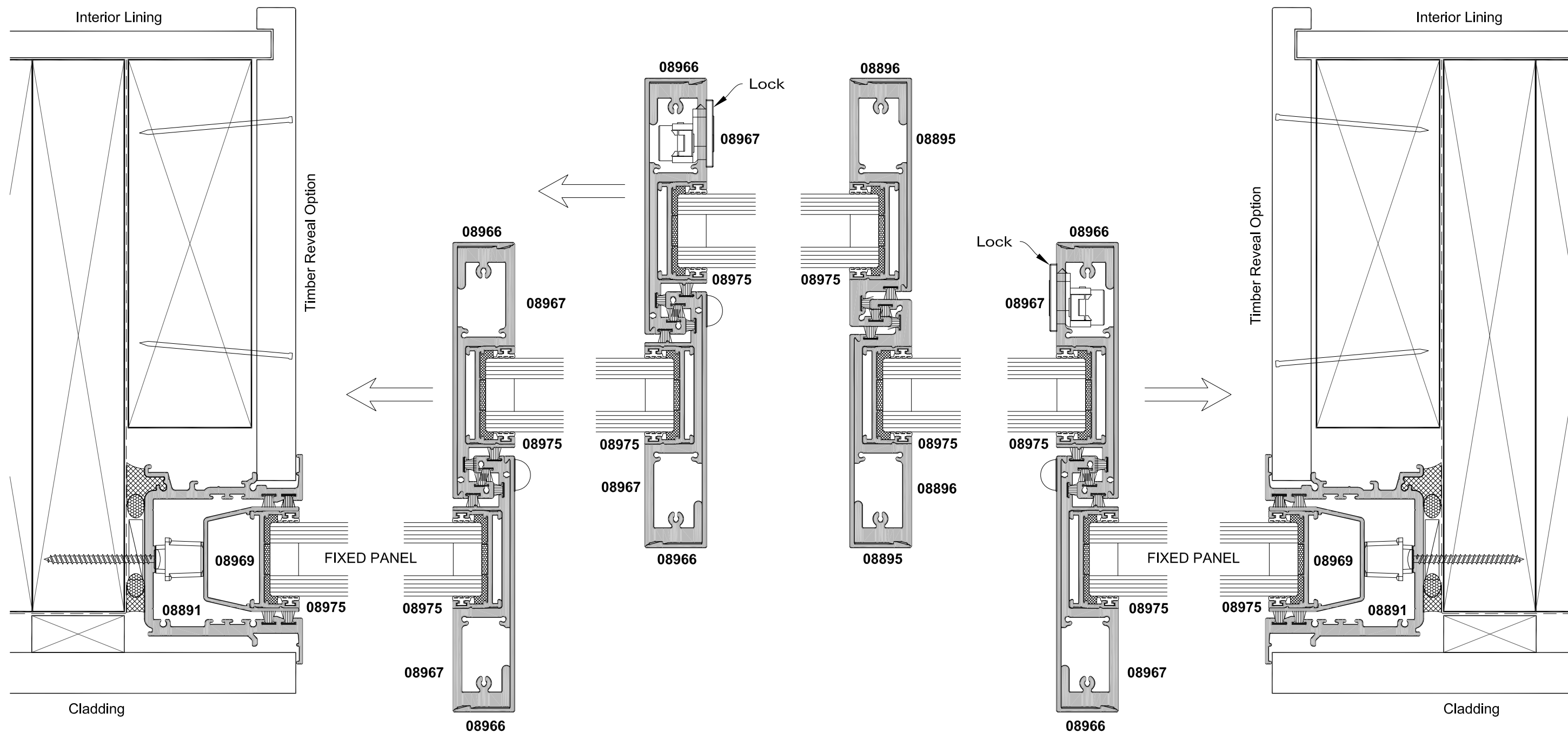
SECTION A-A
