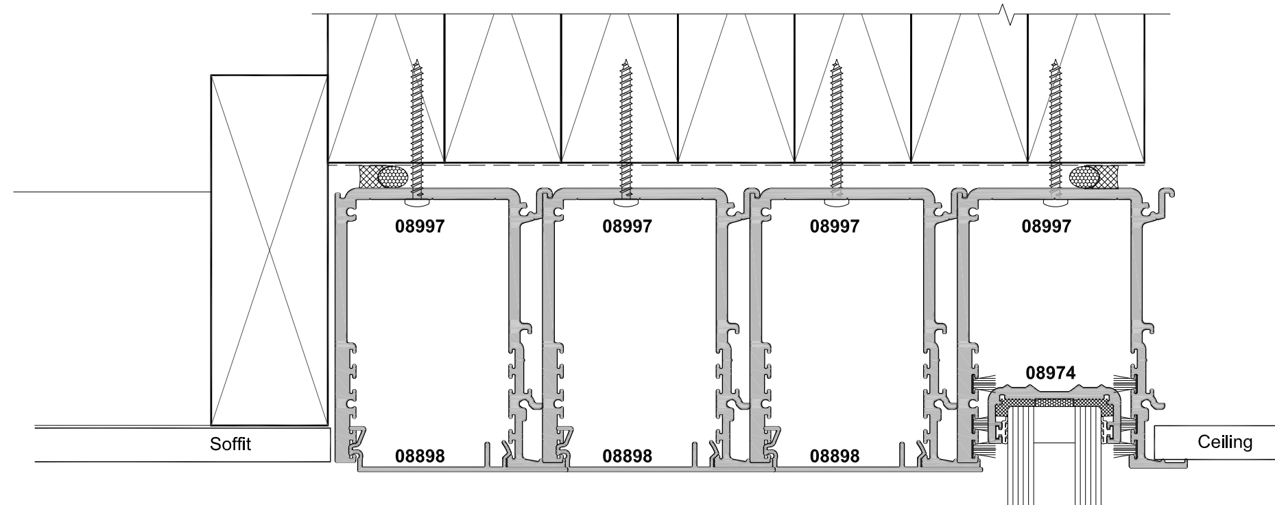
SECTION A-A
