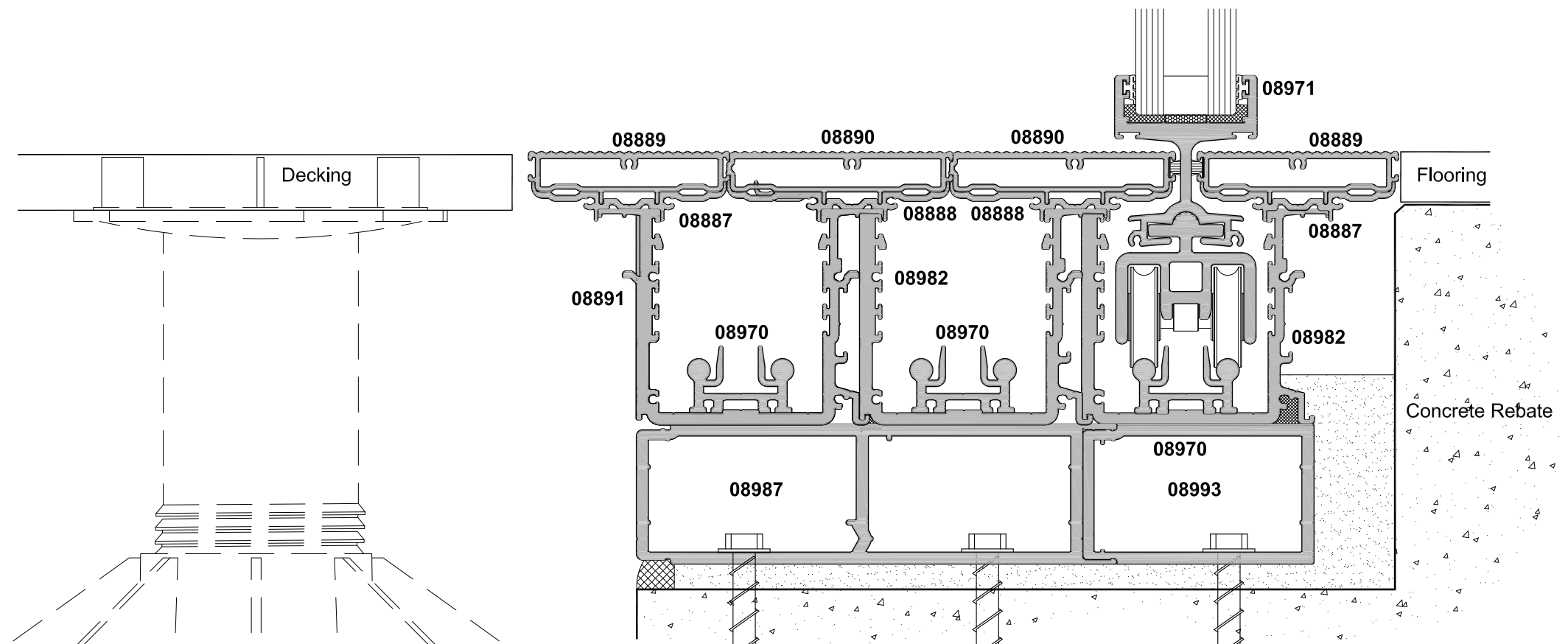
SECTION A-A
