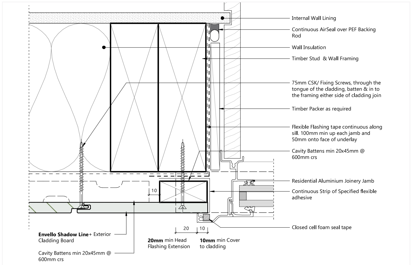
FIG. 20 - WINDOW JAMB
