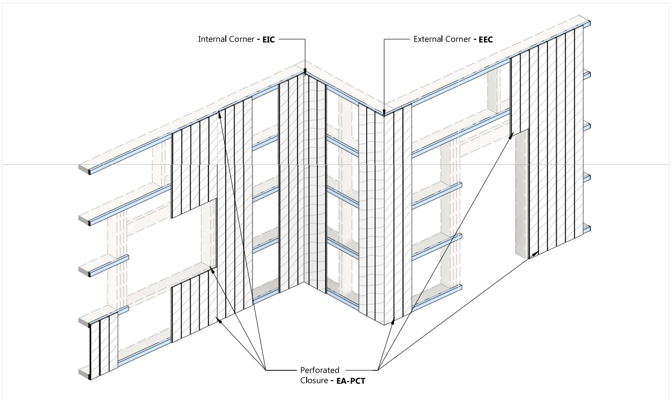
FIG 2 - BATTEN LAYOUT
