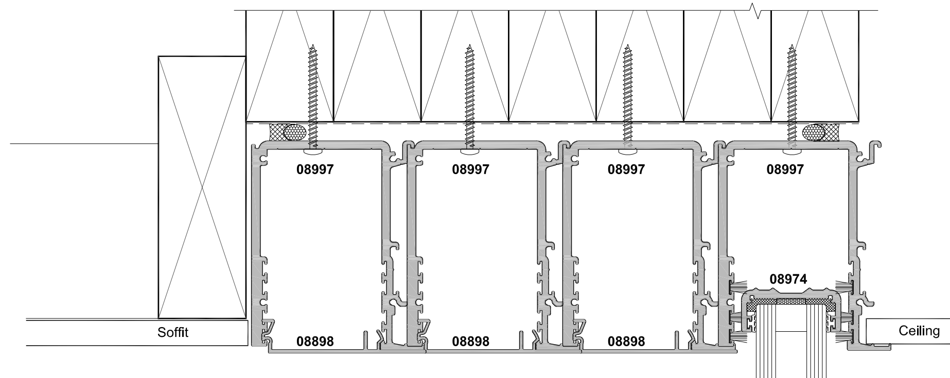
SECTION A-A
