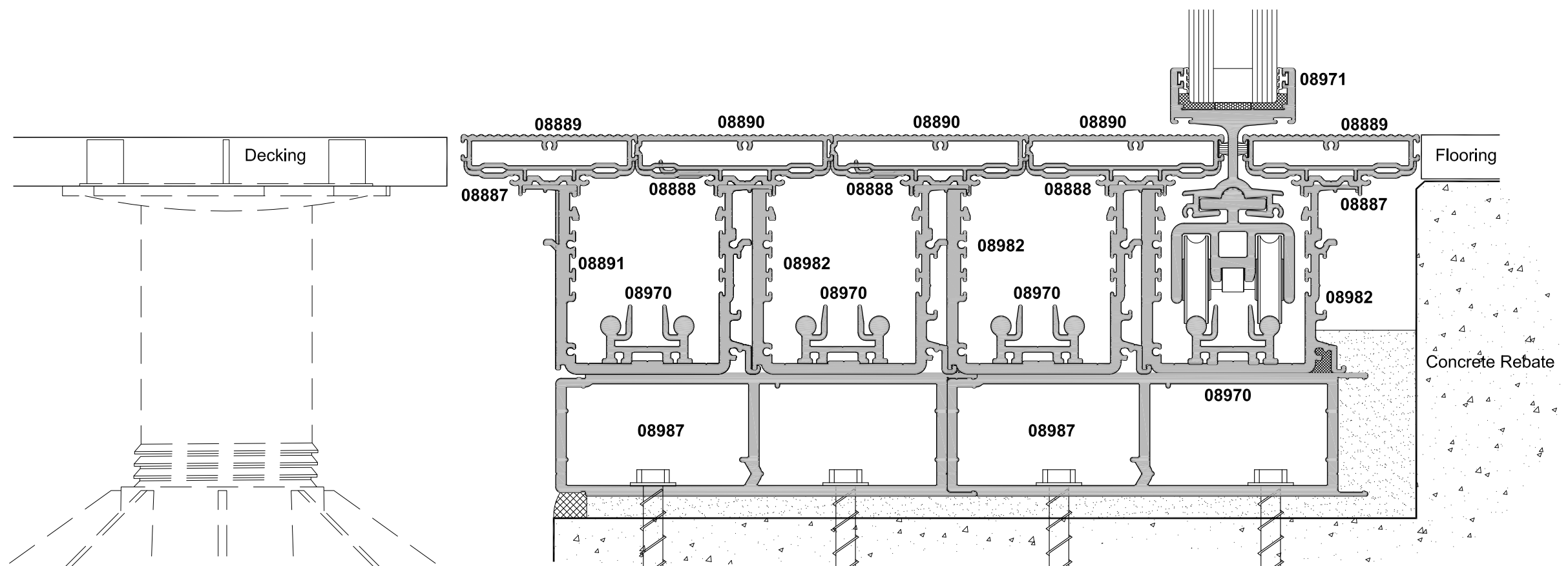
SECTION A-A
